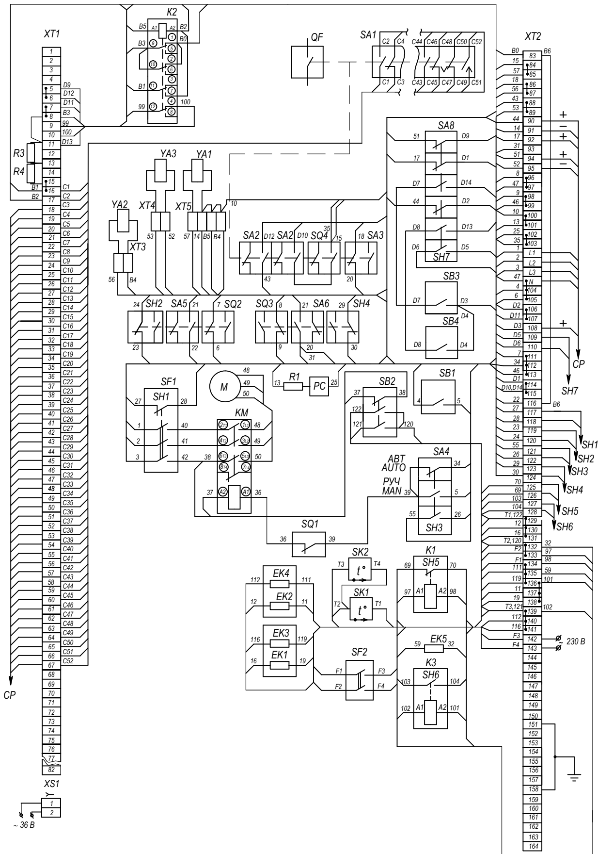
а - исполнение с питанием двигателя от сети U_n=400\text{ В}
