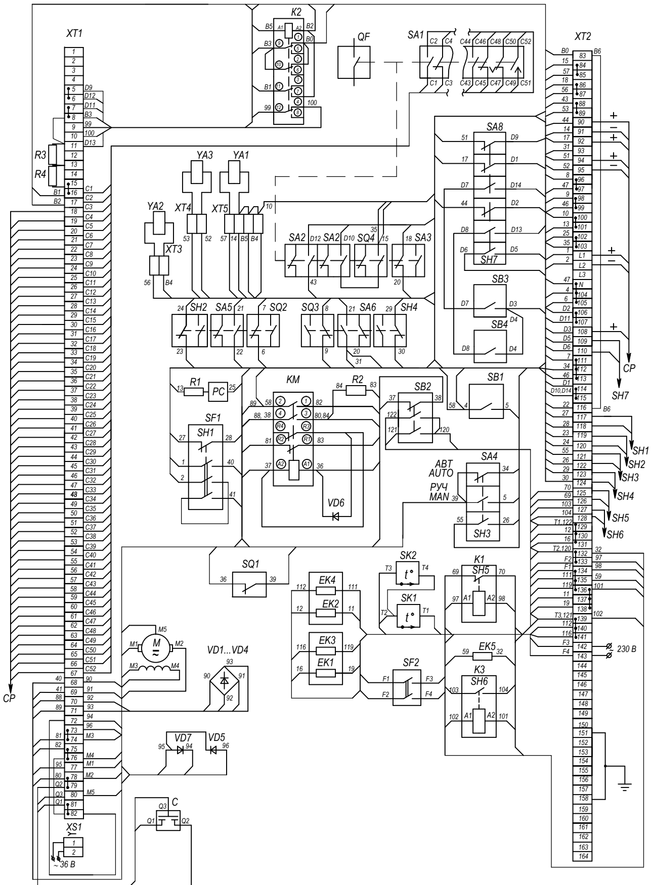
а - исполнение с питанием универсального двигателя от сети: 1. U_n = 230 \text{ В} однофазного переменного тока; 2. 220 \text{ В} (или 110 \text{ В} ) постоянного тока.
