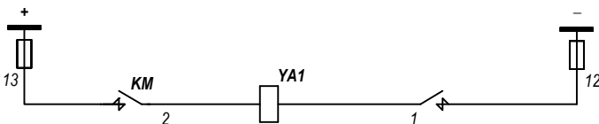
Рисунок 5. Схема электрическая соединений и принципиальная привода ПЭМ-1 (УХЛ1)
