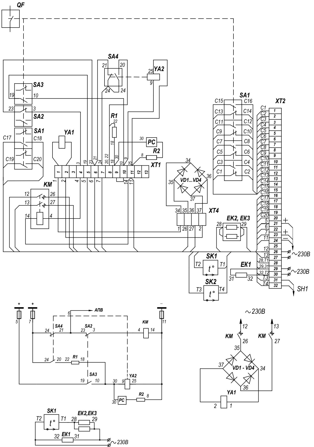
Рисунок 6. Схема электрическая соединений и принципиальная привода ПЭМ-2 (УХЛ1)
