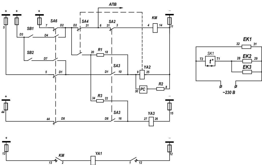
Рисунок 8. Схема электрическая соединений и принципиальная привода ПЭМ-4 (УХЛ1)
